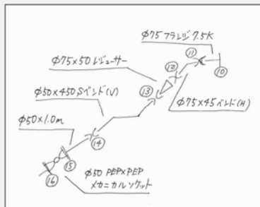
【手書き配管図】
